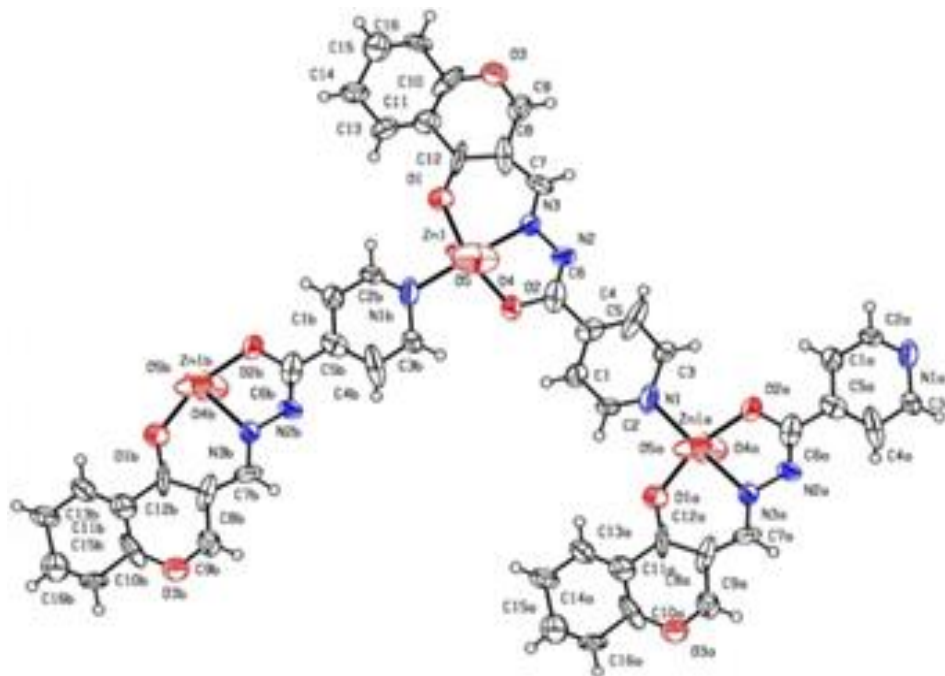
Fig. 1. ORTEP diagram
